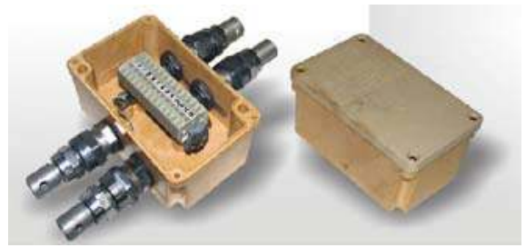
КП-8-00-(1)-10-00-Б2Г2-Г1/2-06-01-11
